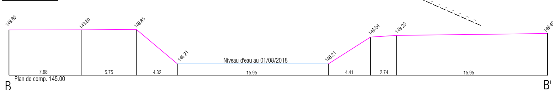
PROFIL B-B'
