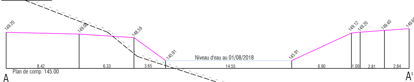
PROFIL A-A'
